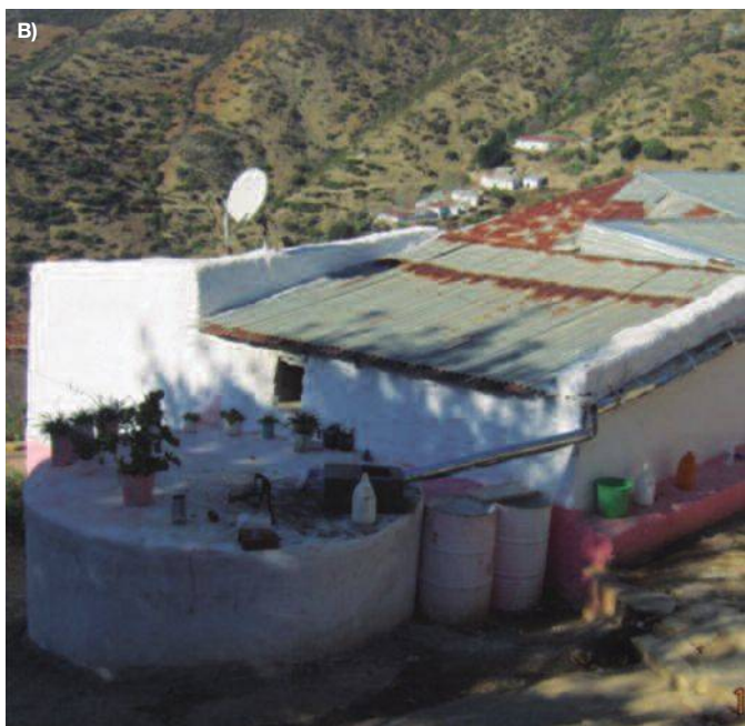
A) Dispositif de captage des eaux pluviales : canalisations, citerne et pompe. B) Captage des eaux pluviales : toiture, gouttière et réservoir.
